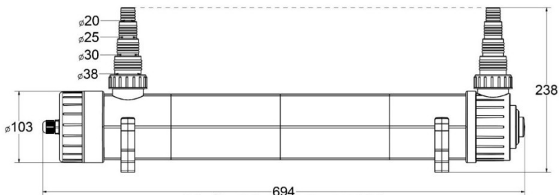
Rys. 4: Wymiary Helix Max 36 W
