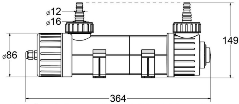
Rys. 2: Wymiary Helix Max 5 - 11 W
