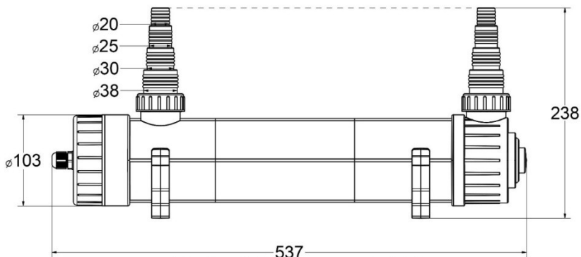
Helix Max 2.0 - 36W
