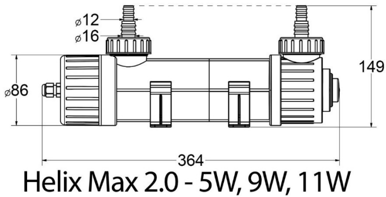
Fig. 2: Dimensiones Helix Max 5 - 11 W
