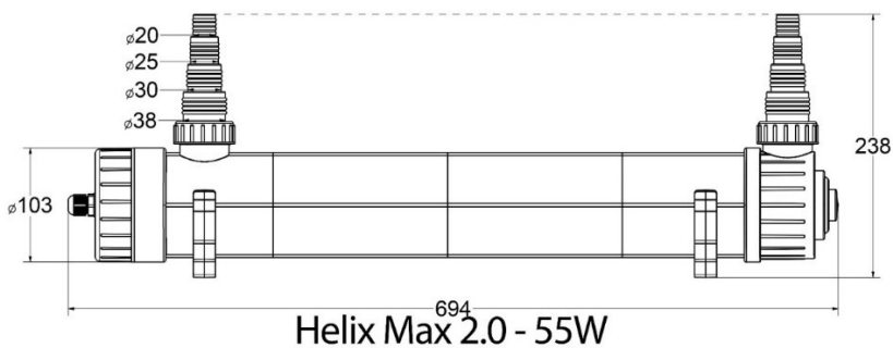
Fig. 5: Dimensioni Helix Max 55 W
