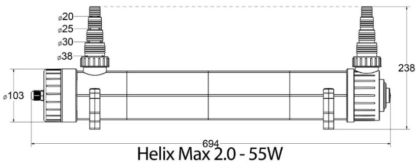
Fig. 5: Dimensiones Helix Max 55 W
