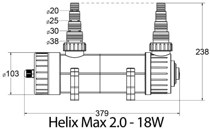
Fig. 3 Dimensions Helix Max 18 W
