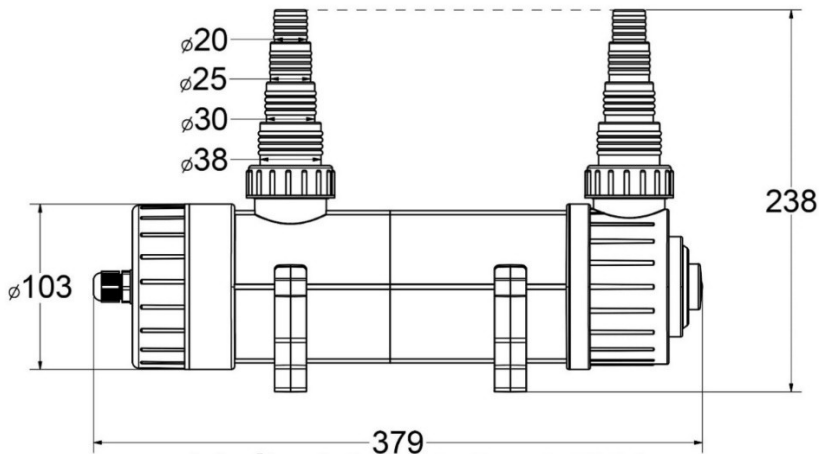
Abb. 2: Abmessungen Helix Max 5 - 11 W
