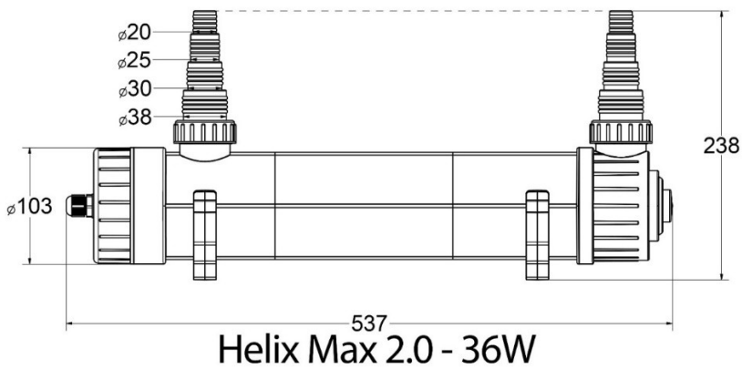
Fig. 4: Dimensiones Helix Max 36 W
