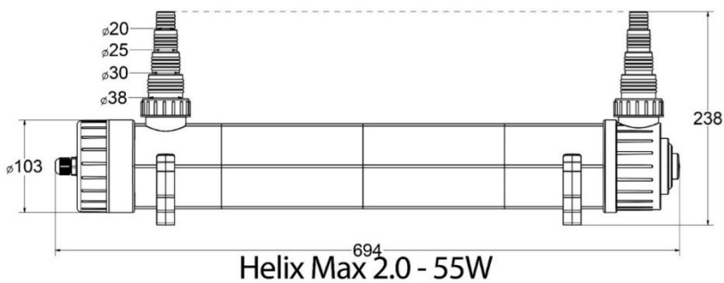
Abb. 5: Abmessungen Helix Max 55 W
