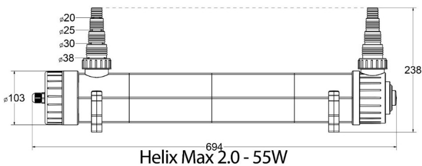
Fig. 5: Dimensions Helix Max 55 W
