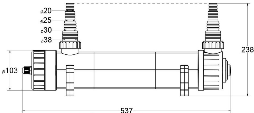
Abb. 3: Abmessungen Helix Max 18 W
