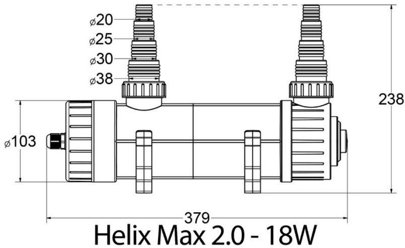
Fig. 3: Dimensiones Helix Max 18 W
