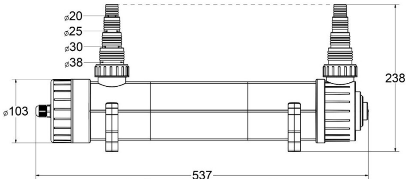
Rys. 3: Wymiary Helix Max 18 W
